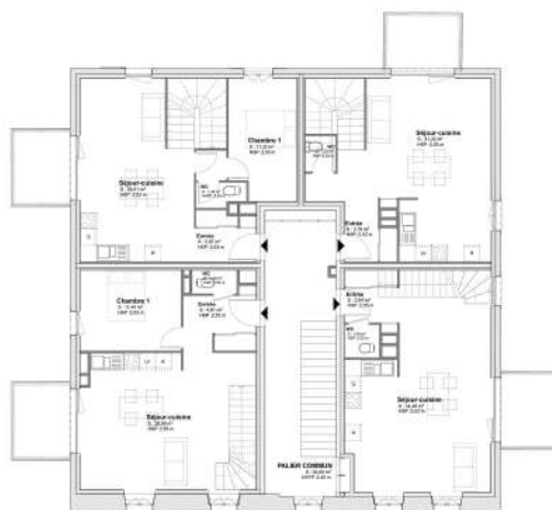
Etage 1
