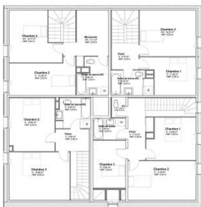
Etage 2 (duplex)
